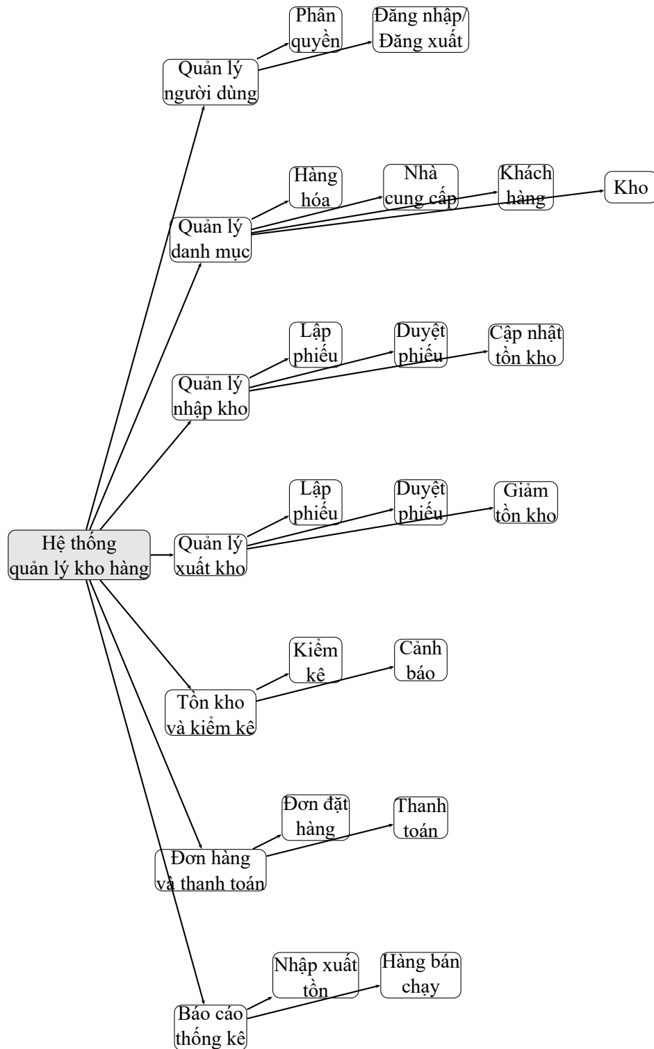
Hình 3.1: Sơ đồ phân cấp chức năng (BFD) hệ thống quản lý kho hàng
