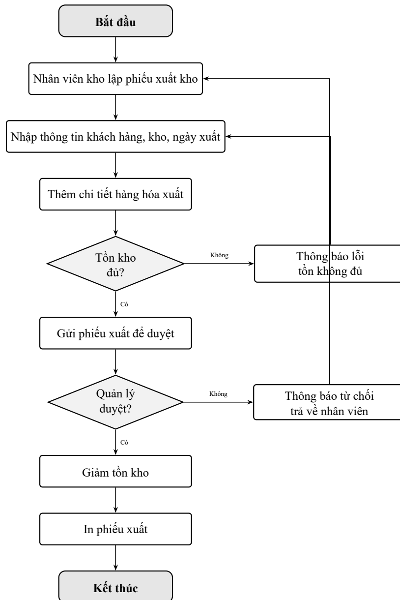
Hình 2.2: Sơ đồ hoạt động quy trình xuất kho
