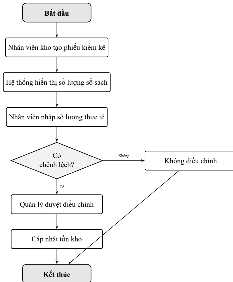
Hình 2.3: Sơ đồ hoạt động quy trình kiểm kê tồn kho
