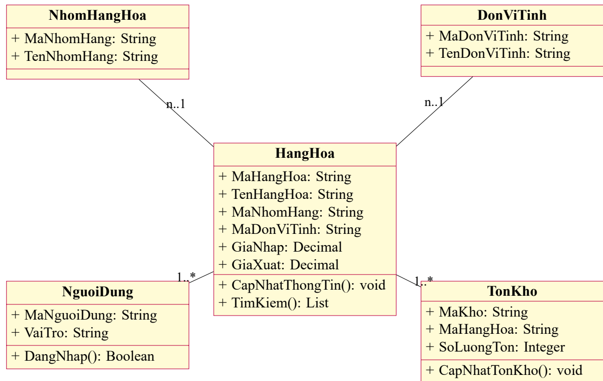
Hình 4.4: Biểu đồ lớp trong ca sử dụng UC05 – Quản lý hàng hóa
