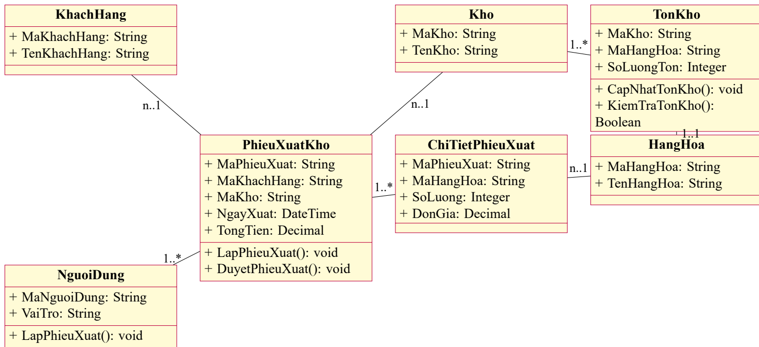
Hình 4.6: Biểu đồ lớp trong ca sử dụng UC10 – Lập phiếu xuất kho
