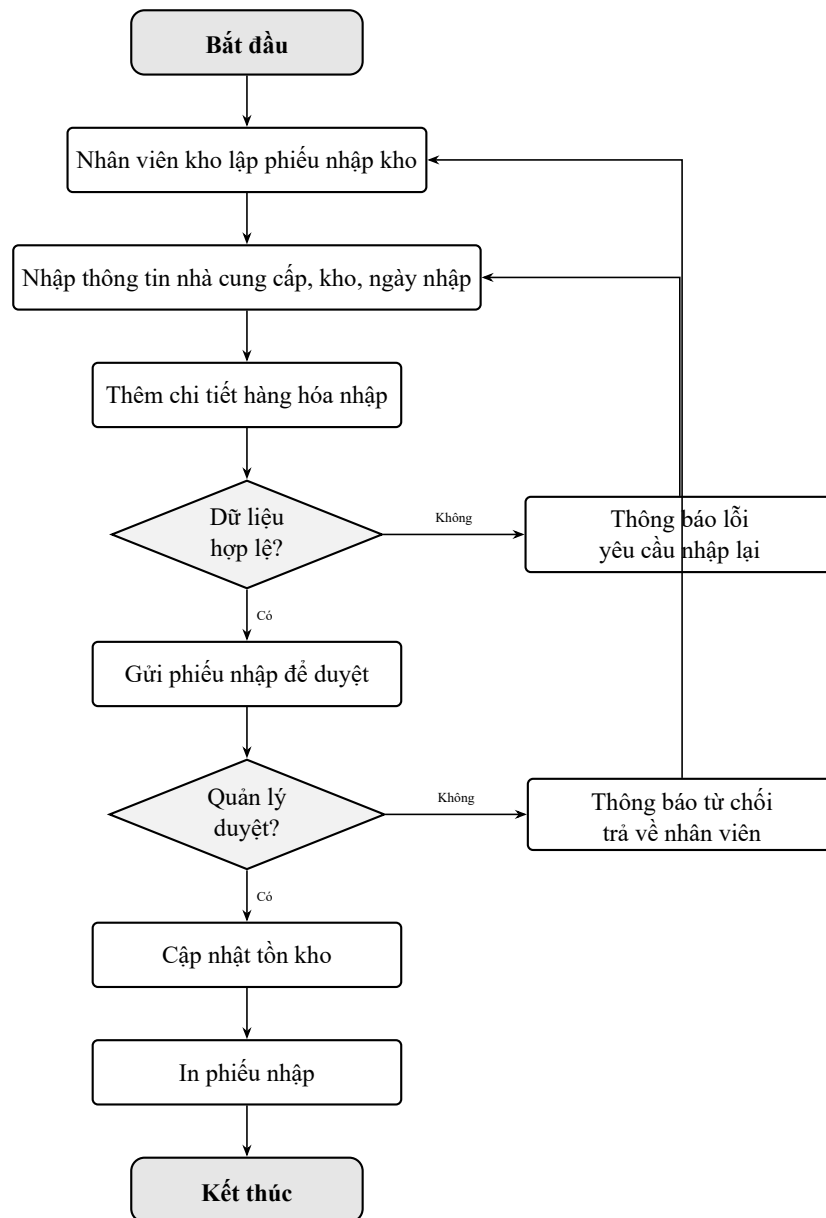
Hình 2.1: Sơ đồ hoạt động quy trình nhập kho
